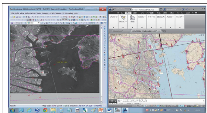
ALOS-1 衛星ステレオ画像とGCPs基準点と1秒毎の運動経路 ALOS-1 satellite stereo images and DGPS-GCPs with 1 second interval positioning
