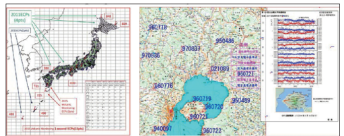
2011年-2015年—全国与点電子基準点と鹿児島桜島周辺観測局 2011-2015—national network adjustment and Sakurajima project (volcanic eruption)
